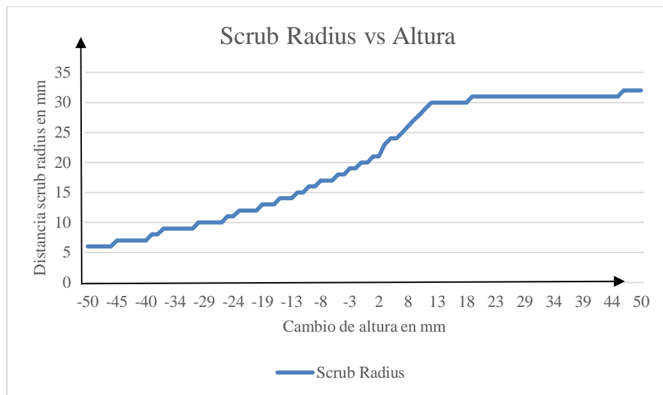
Figura 3.33 Scrub radius trasero vs altura chasis Fuente: Elaboración propia
