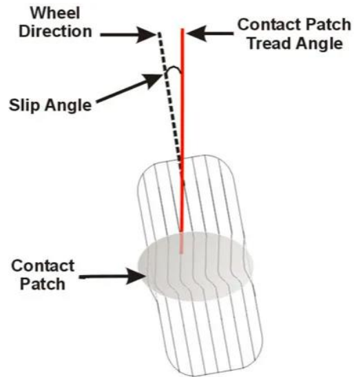
Figura 1.14 Slip Angle Fuente: Suspension Secrets [19]
