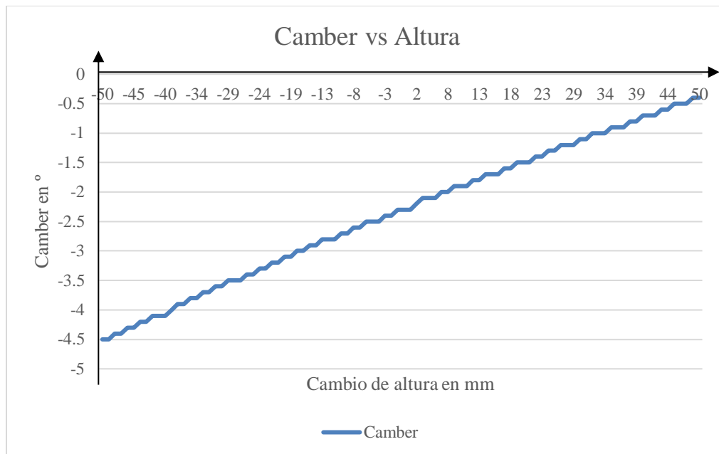
Figura 3.18. Camber vs altura chasis Fuente: Elaboración propia
