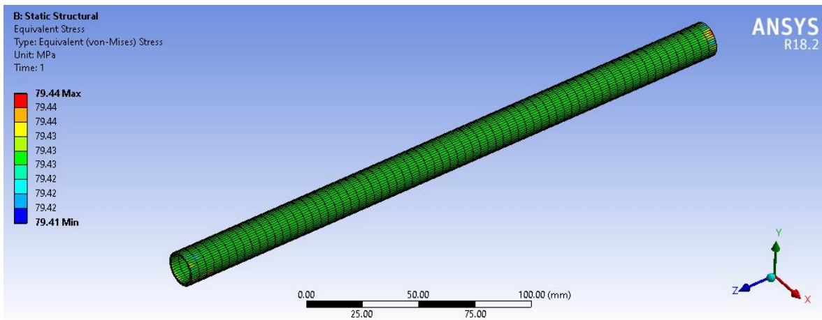
Figura 3.42 Esfuerzos varilla de empuje delantera Fuente: Elaboración propia desde ANSYS
