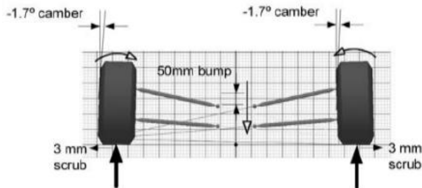
Figura 2.6 Brazos de igual longitud no-paralelos en movimiento vertical Fuente: Race Car Design Derek Seward [13]
