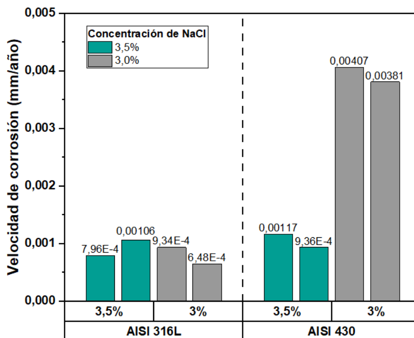
Figura 3.8 Esquema de las velocidades de corrosión de los aceros inoxidables AISI 316L y AISI 430 en solución de NaCl 3.5% y 3.0% Fuente: Elaboración propia
