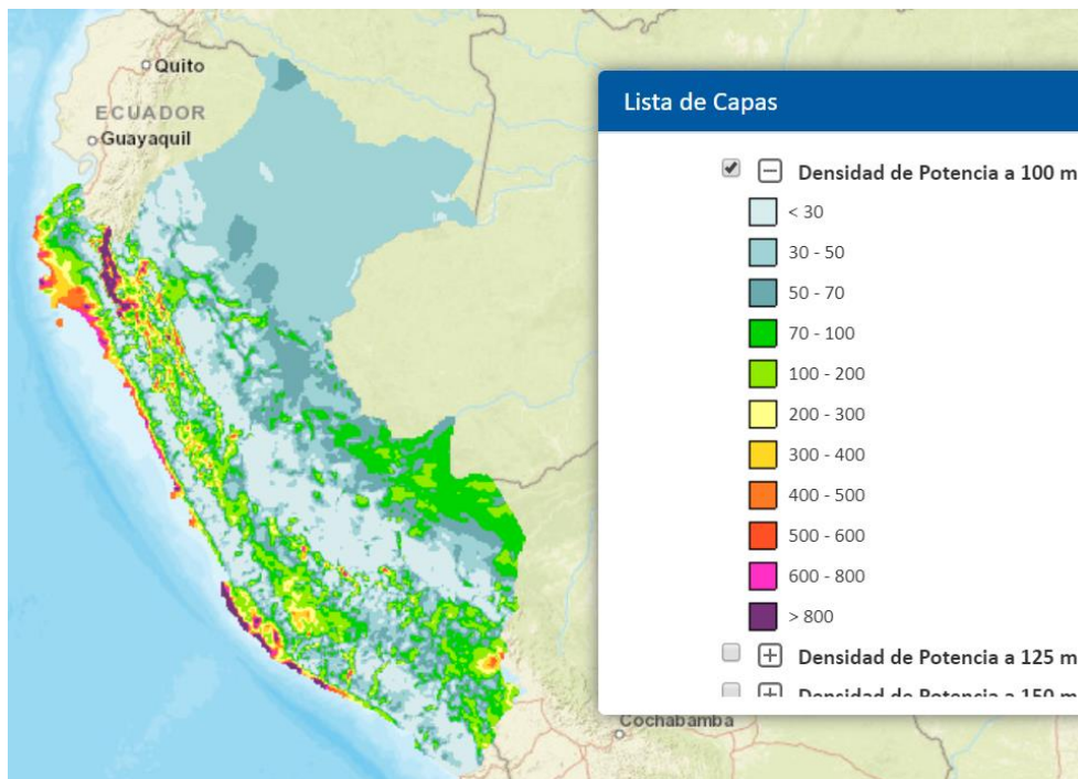
Figura 3.4 Ubicación geográfica del potencial eólico del Perú a 100m promedio anual Fuente: Osinermin, Mapa Energético Minero [65]
