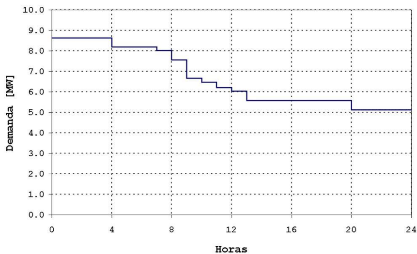
Figura 1.6 Curva de duración de carga
