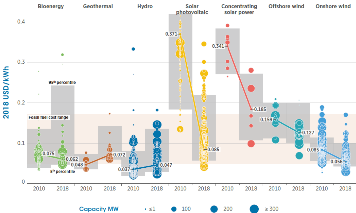
Figura 1.13 LCOE global de plantas de energía renovable de gran escala, 2010-2018 Fuente: IRENA. Costos de Generación Eléctrica de Energía Renovable en 2018. [38]
