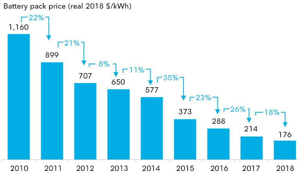
Figura 1.17 Resultados de la entrevista de precio de baterías de litio de BloombergNEF Fuente: BloombergNEF. A Behind the Scenes Take on Lithium-ion Battery Prices [55].
