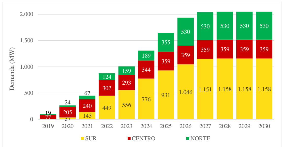
Figura 4.2 Demanda proyectada por zona geográfica Fuente: Elaboración propia
