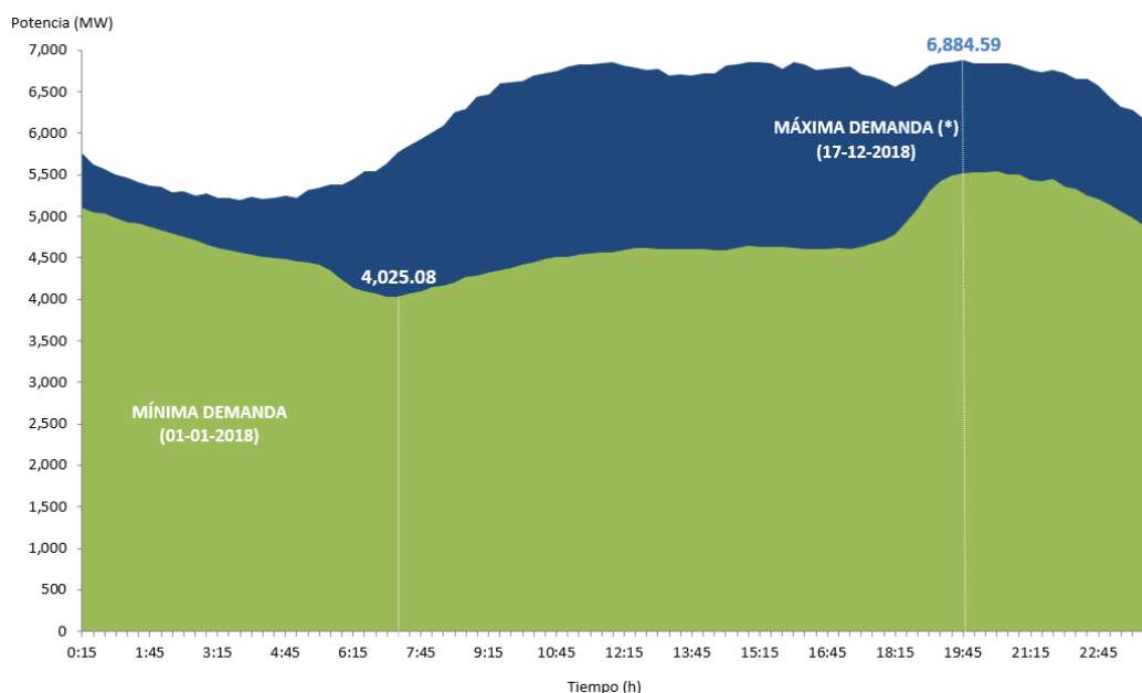
Figura 1.12 Perfil de carga del día de la mínima y máxima demanda del SEIN 2018 Fuente: COES. Estadística anual 2018 [37]
