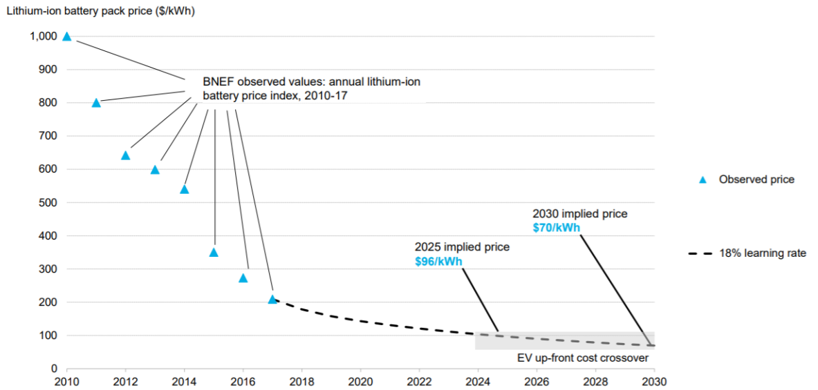
Figura 1.19 Proyección de precio de baterías de litio de BloombergNEF Fuente: BloombergNEF. A Behind the Scenes Take on Lithium-ion Battery Prices [55].
