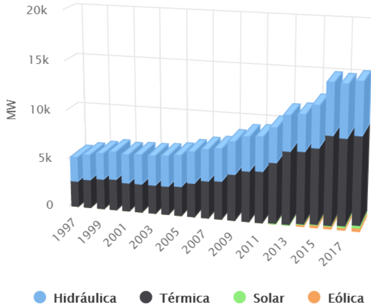
Figura 1.8 Evolución de la potencia instalada nacional Fuente: Osinergmin. Observatorio Energético Mínero [34]
