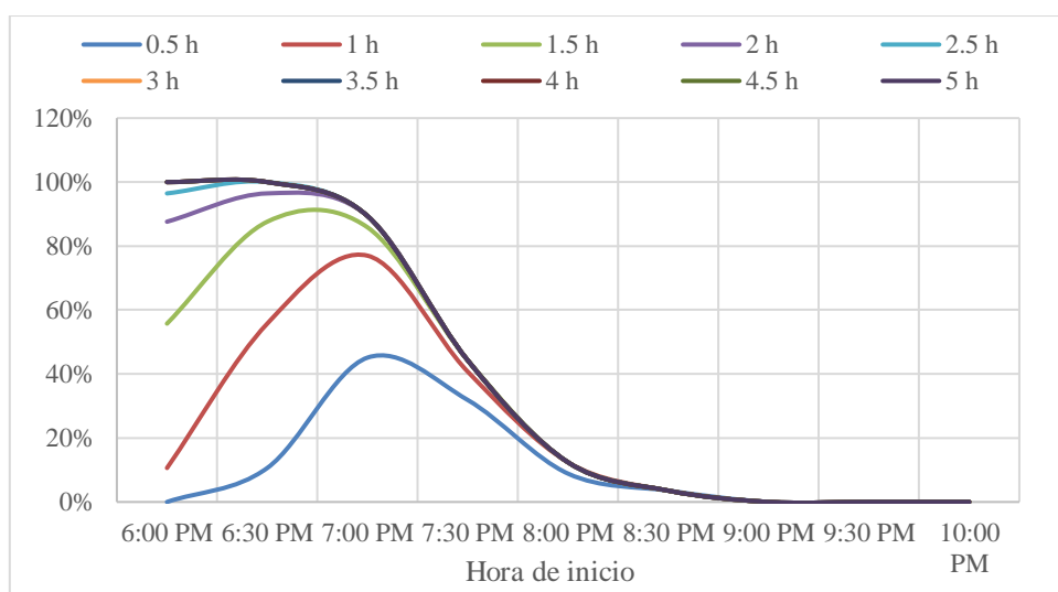
Figura 4.9 Nivel de incidencia de la máxima demanda del SEIN, según hora de inicio de descarga y duración de la batería Fuente: elaboración propia
