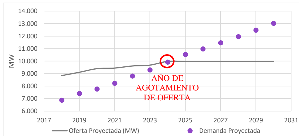
Figura 4.4 Superposición de las proyecciones de oferta y demanda eléctrica Fuente: Elaboración propia
