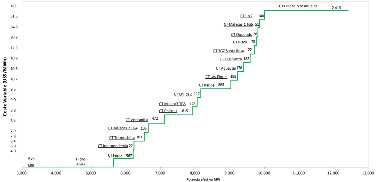
Figura 1.2 Curva de oferta de eléctrica Fuente: Laub & Quijandría. Reporte del Mercado Eléctrico [27]
