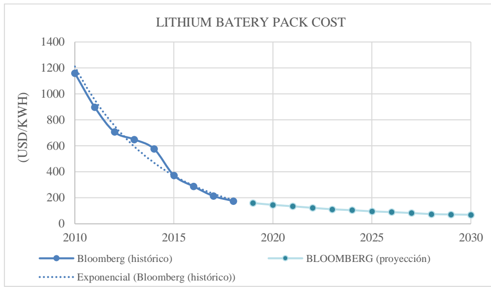
Figura 4.8 Proyección de costos capitales para las baterías de litio Fuente: Bloomberg NEF, A Behind the Scenes Take on Lithium-ion Battery Prices [55]
