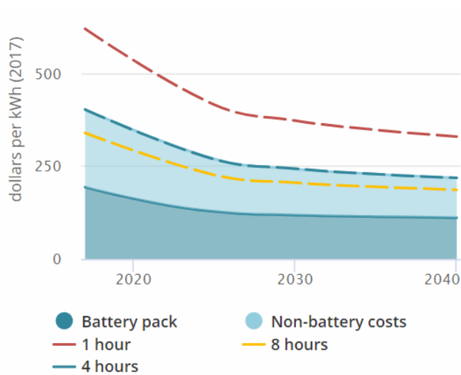
Figura 1.20 Proyección de precio de baterías de litio de International Energy Agency (IEA) Fuente: IEA. Costs of utility-scale battery storage systems in the New Policies Scenario [57].
