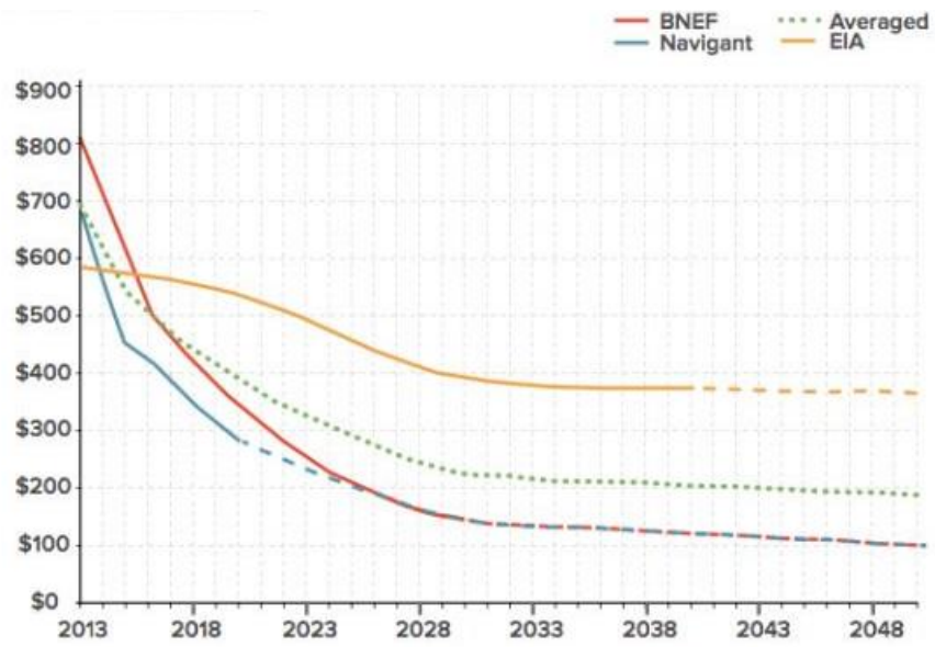
Figura 1.21 Comparación de proyecciones de baterías de litio de Rocky Mountain Institute (RMI) Fuente: Greentech Media / RMI. Storage is the New Solar: Will Batteries and PV Create an Unstoppable Hybrid Force? [58].
