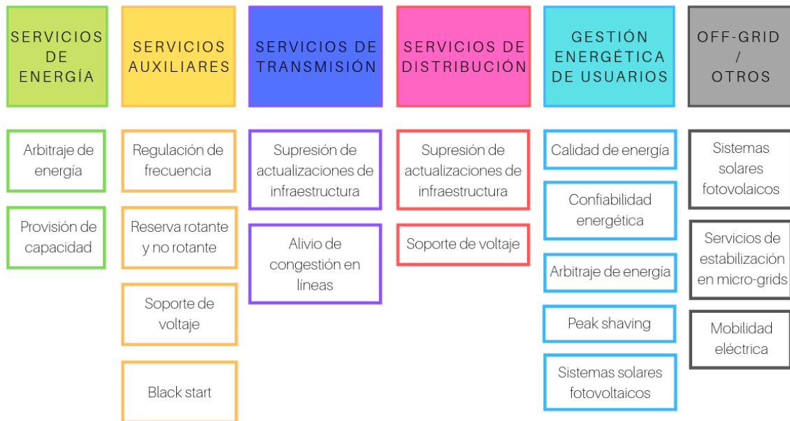
Figura 1.16 El rango de servicios que puede proveer el almacenamiento eléctrico Fuente: IRENA. Electricity Storage a Renewables: Costs and Markets to 2030 [43]
