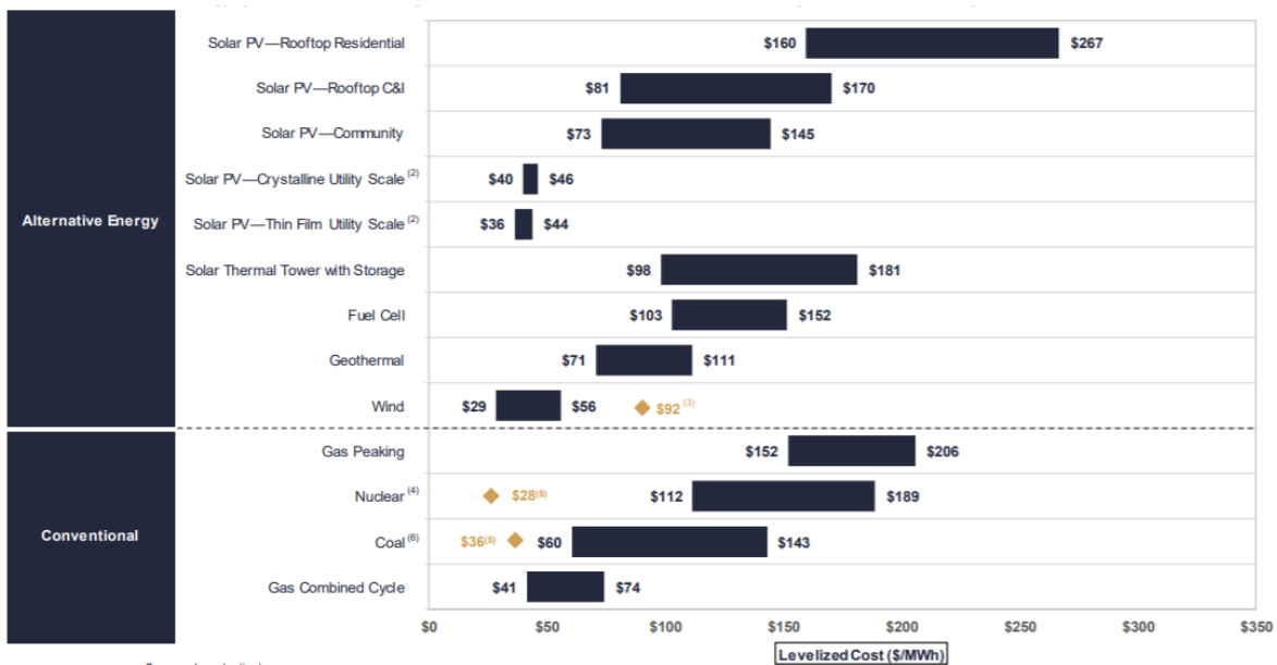
Figura 1.14 LCOE global de distintas tecnologías de generación al 2018 Fuente: Lazard. Análisis de Costos Nivelados de Electricidad de Lazard – Versión 12.0 [39]
