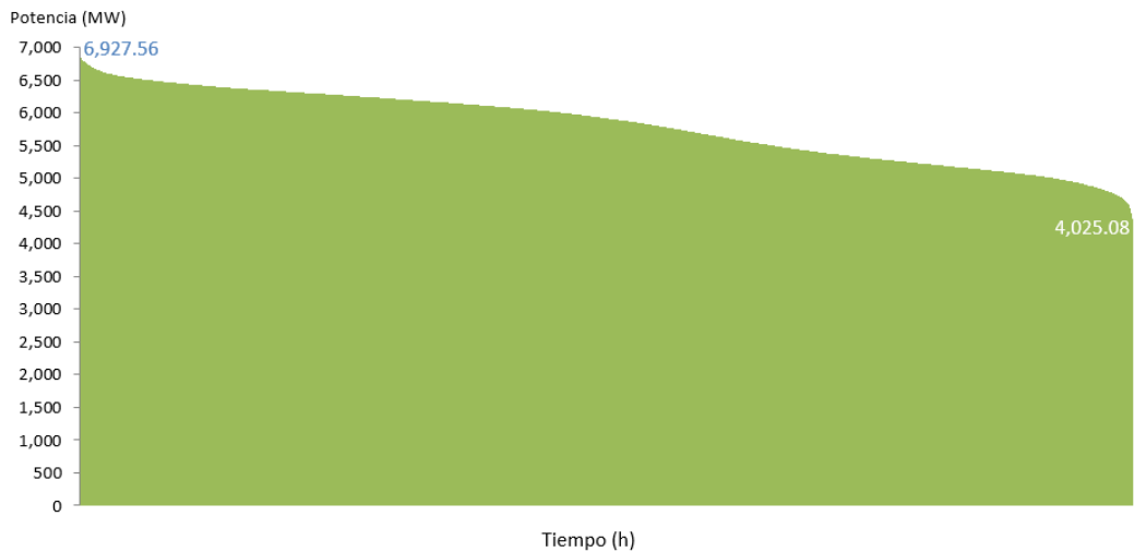
Figura 1.11 Curva de duración de carga 2018 Fuente: COES. Estadística anual 2018 [37]
