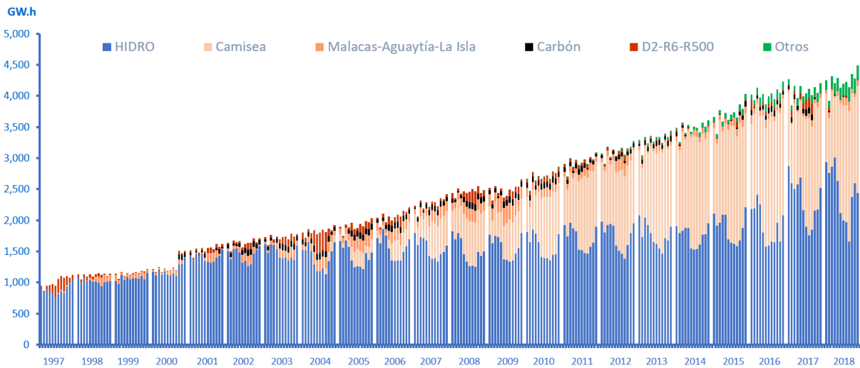
Figura 1.10 Evolución de la producción eléctrica según tipo de generación Fuente: COES. Estadística anual 2018 [36]
