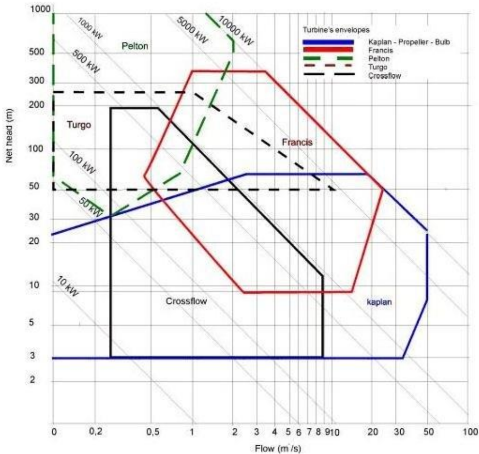
Figura 1.15 Diagrama de selección de turbina según flujo y altura
