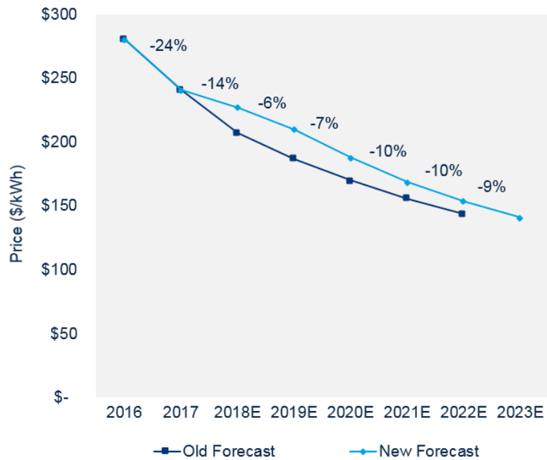
Figura 1.18 Proyección de precio de baterías de litio de Wood Mackenzie Fuente: Wood Mackenzie Power & Renewables. Battery Rack Price Forecast, 2016-2023E ($/kWh) [56].
