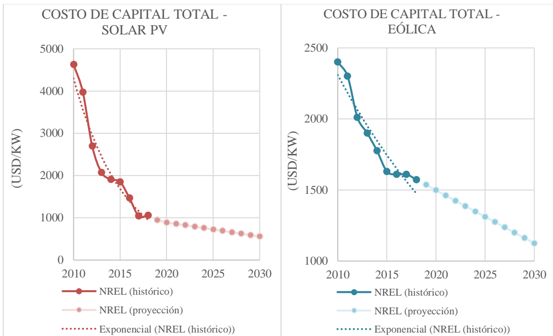
Figura 4.7 Proyecciones de costos capitales para las tecnologías solar y eólica, escenario optimista Fuente: NREL, Línea Base Anual de Tecnología de Electricidad del 2019 [77]
