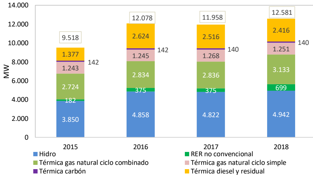
Figura 1.3 Evolución de la potencia efectiva del parque generador del Perú 2015-2018 Fuente: COES. Elaboración: Laub & Quijandría [27]
