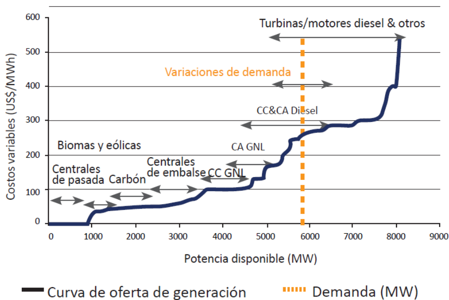
Figura 1.4 Curva de oferta y demanda
