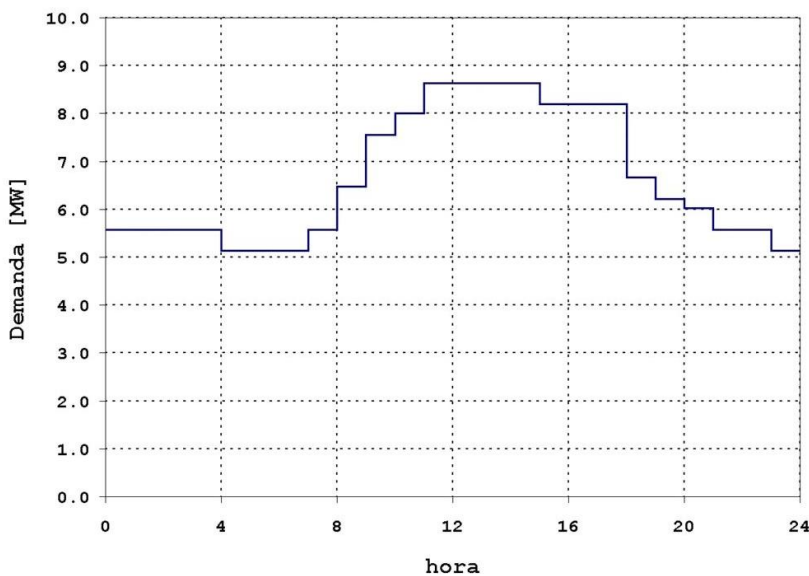
Figura 1.5 Perfil de carga diario
