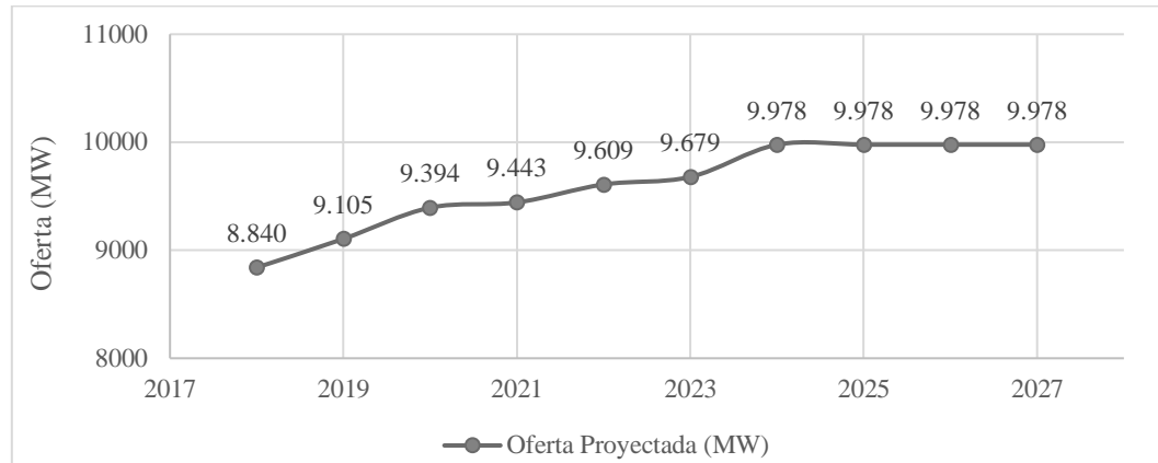
Figura 4.3 Estructuración de la oferta con los proyectos comprometidos Fuente: Elaboración propia
