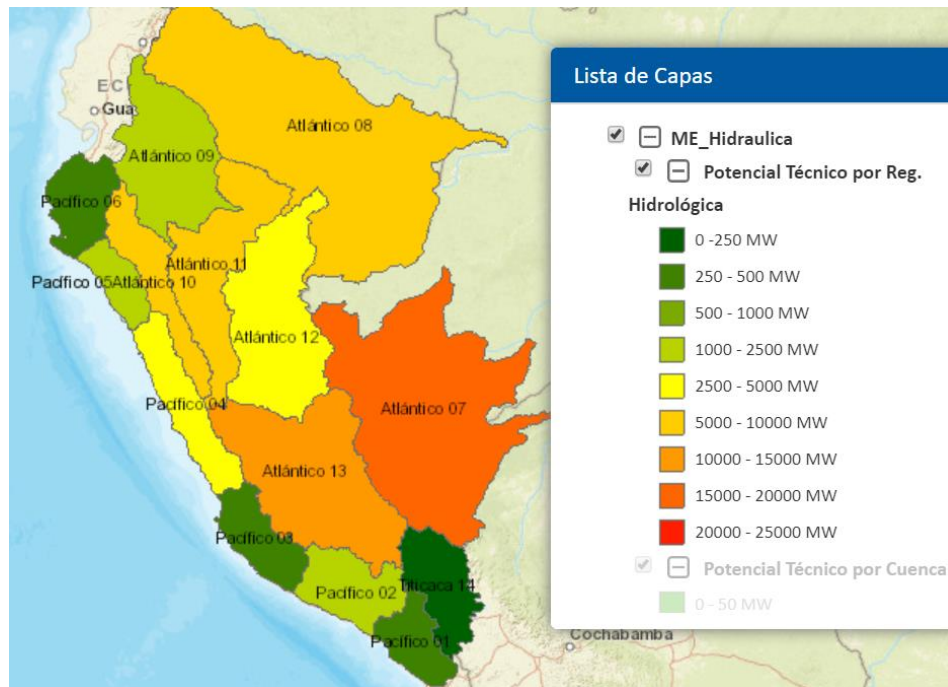
Figura 3.3 Ubicación geográfica del potencial hidroenergético del Perú Fuente: Osinermin, Mapa Energético Minero [65]
