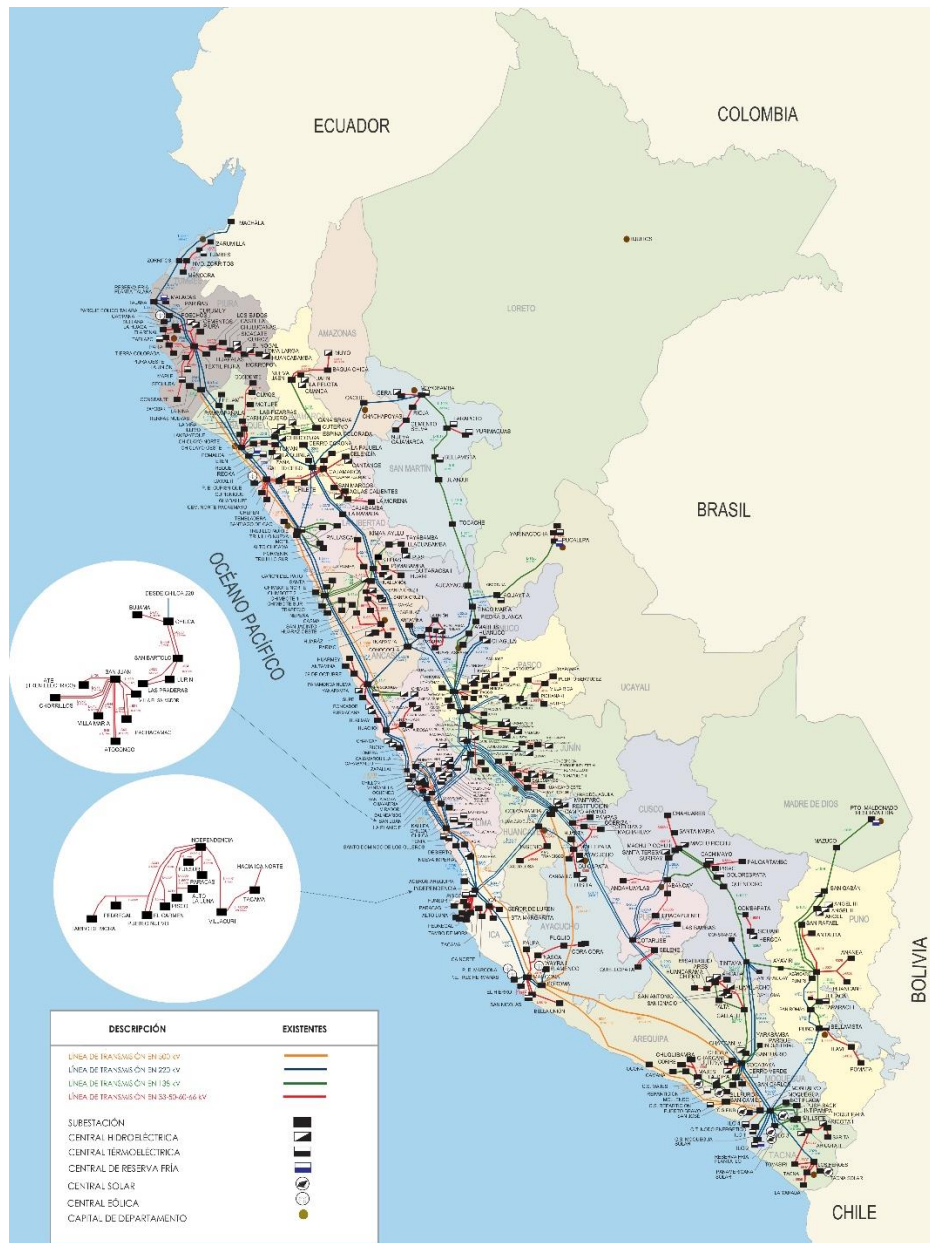
Figura 3.8 Ubicación geográfica de las líneas de transmisión del Perú Fuente: COES, Estadística Anual 2018 [68]
