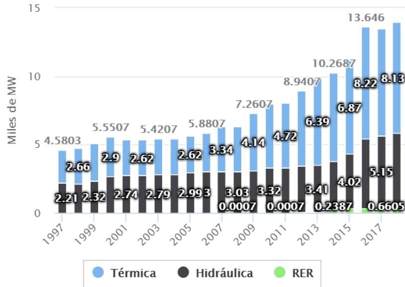
Figura 1.9 Evolución de la potencia efectiva nacional Fuente: Osinergmin. Observatorio Energético Minero [34]
